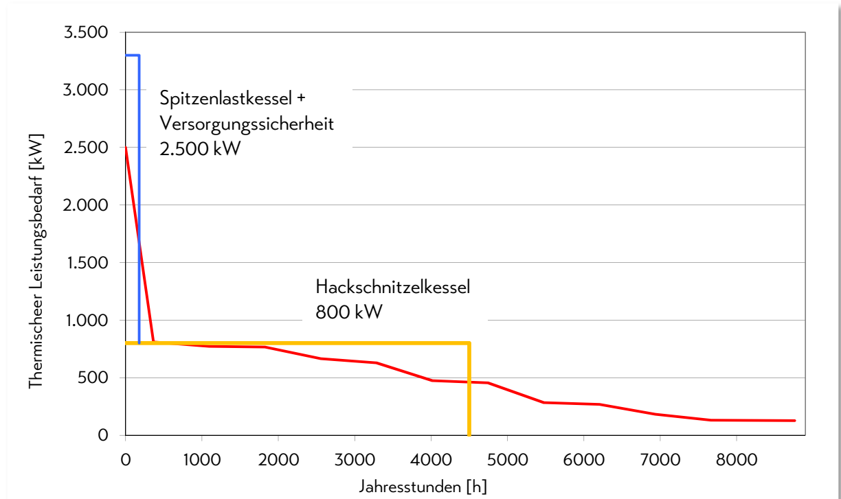
Abbildung 30: Thermische Jahresdauerlinie und eine mögliche Energieversorgungsvariante der Nahwärmeverbundlösung (Szenario 2)
