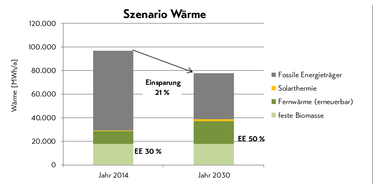
Abbildung 27: Szenario Wärme
