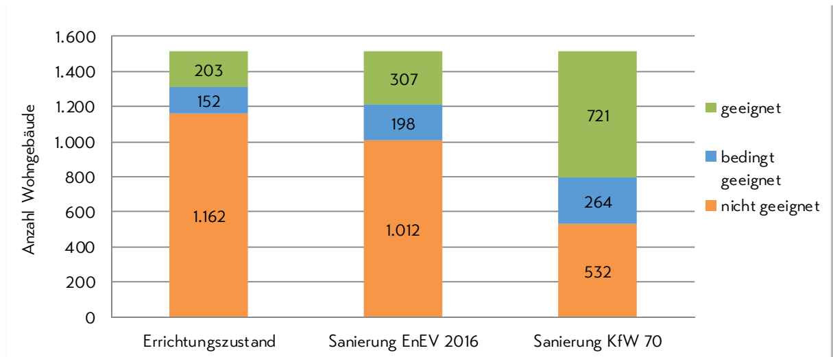
Abbildung 22: Versorgungspotenzial durch Erdwärmesonden in der Gemeinde Bischofswiesen
