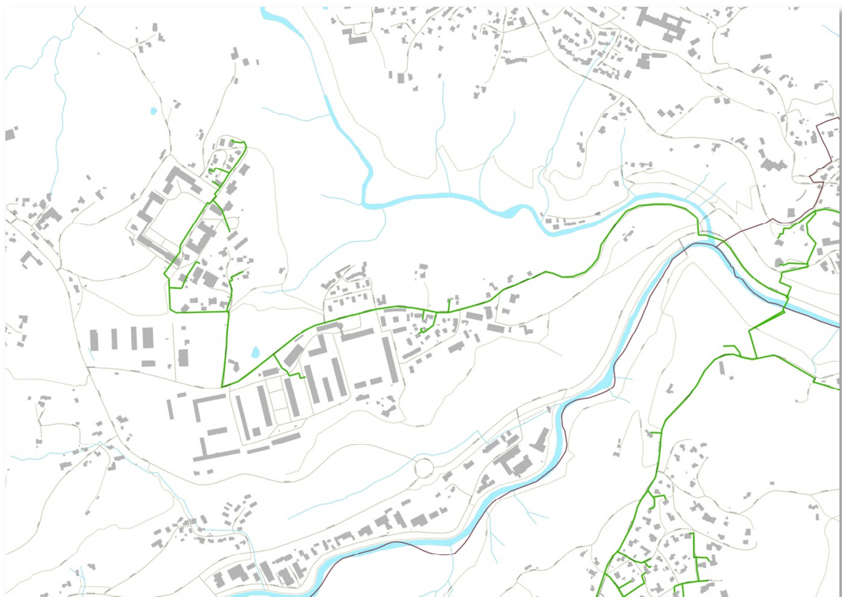
Abbildung 11: Fernwärmeversorgung der Bioenergie Berchtesgadener Land im Ortsteil Strub (Stand 2014)
