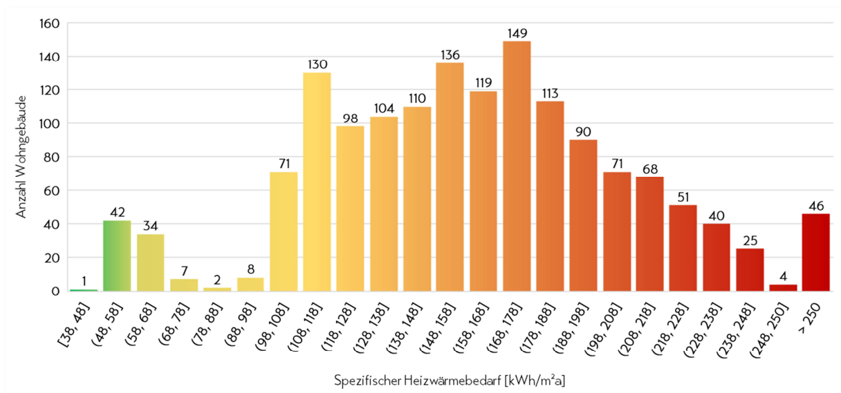
Abbildung 12: Energieeffizienz des Gebäudebestandes in der Gemeinde Bischofswiesen
